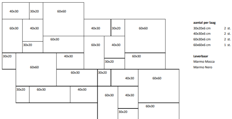
Legvoorbeeld wildverband facetta type 2
